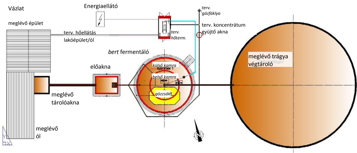
trágyafeldolgozó berendezés egyszerűsített sematikus ábrája a meglévő infrastruktúra használata mellett
